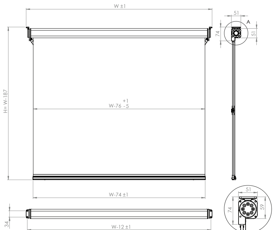
DETTAGLIO A SCALA 1 : 3
